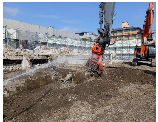
基礎撤去
